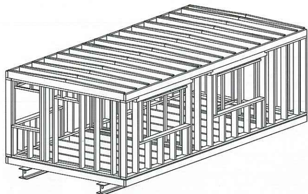
Vue 3D de la structure de l'ossature
